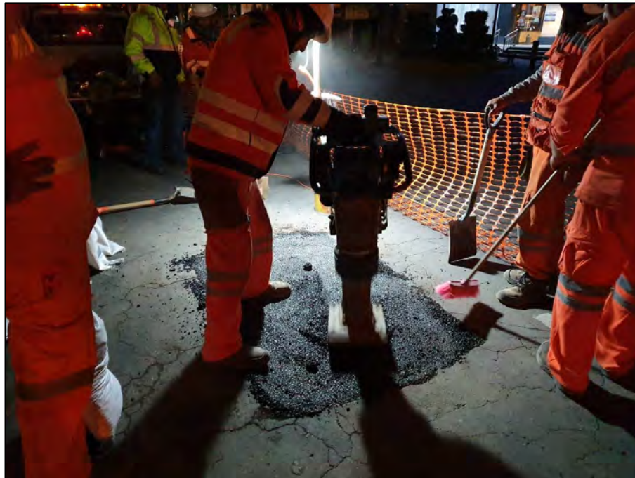
Figura 2.4. Relleno y compactación del PCA
