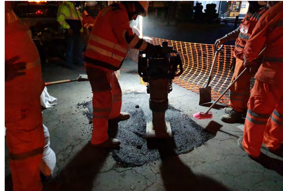
Figura 6. Colocación de asfalto en el PCA-01
