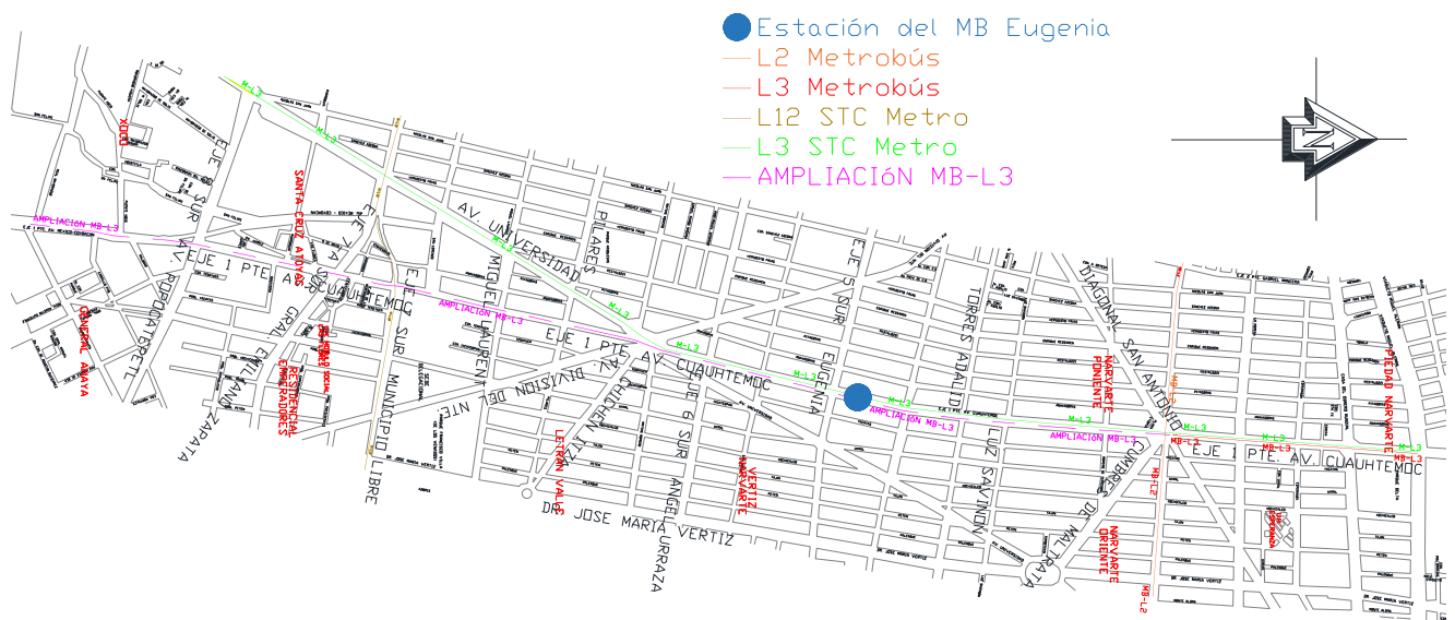
Figura 1.2. Trazo de la ampliación de la Línea 3 del Metrobús y ubicación de la estación Eugenia
