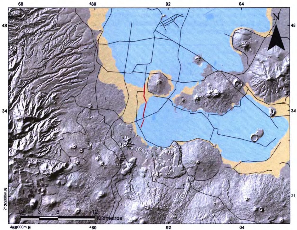
Fig. 8. Trazo del METROBÚS bajo el contexto de la zonificación geotécnica.
