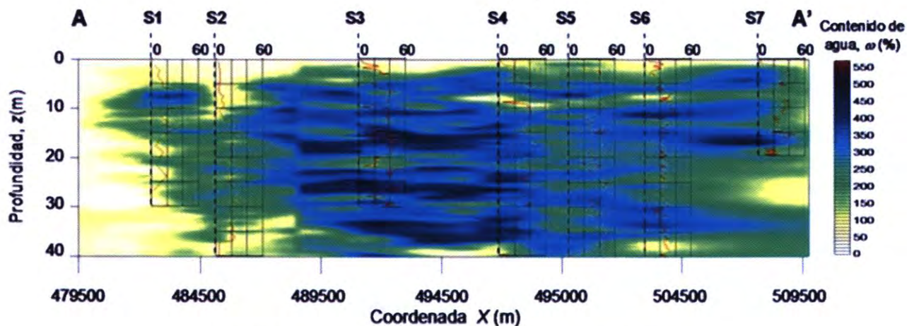
Corte A-A' estimado y sondeos de referencia
