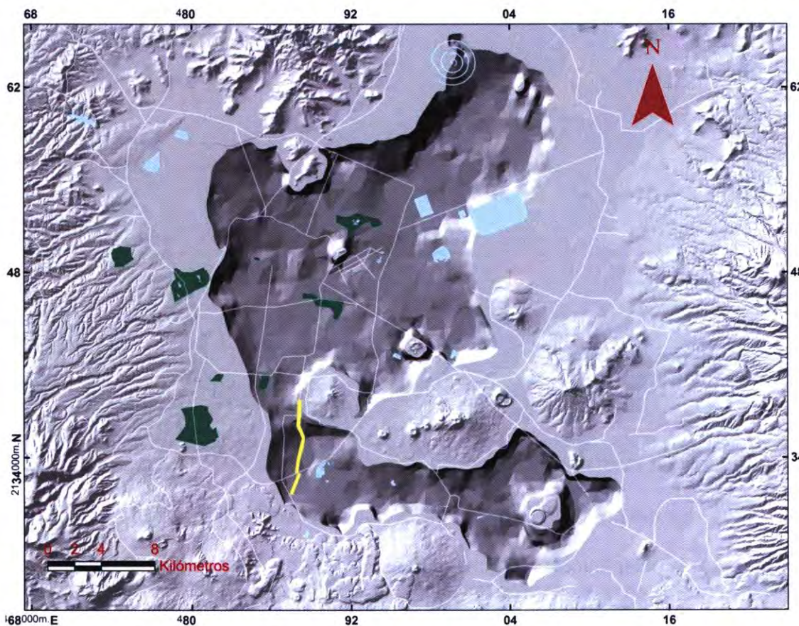
Fig. 19. Hondonada ocasionada por la extracción de agua mediante pozos profundos.
