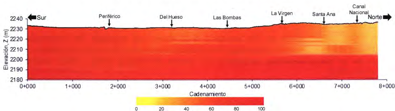
b) Desviación estándar de la estimación (%).
