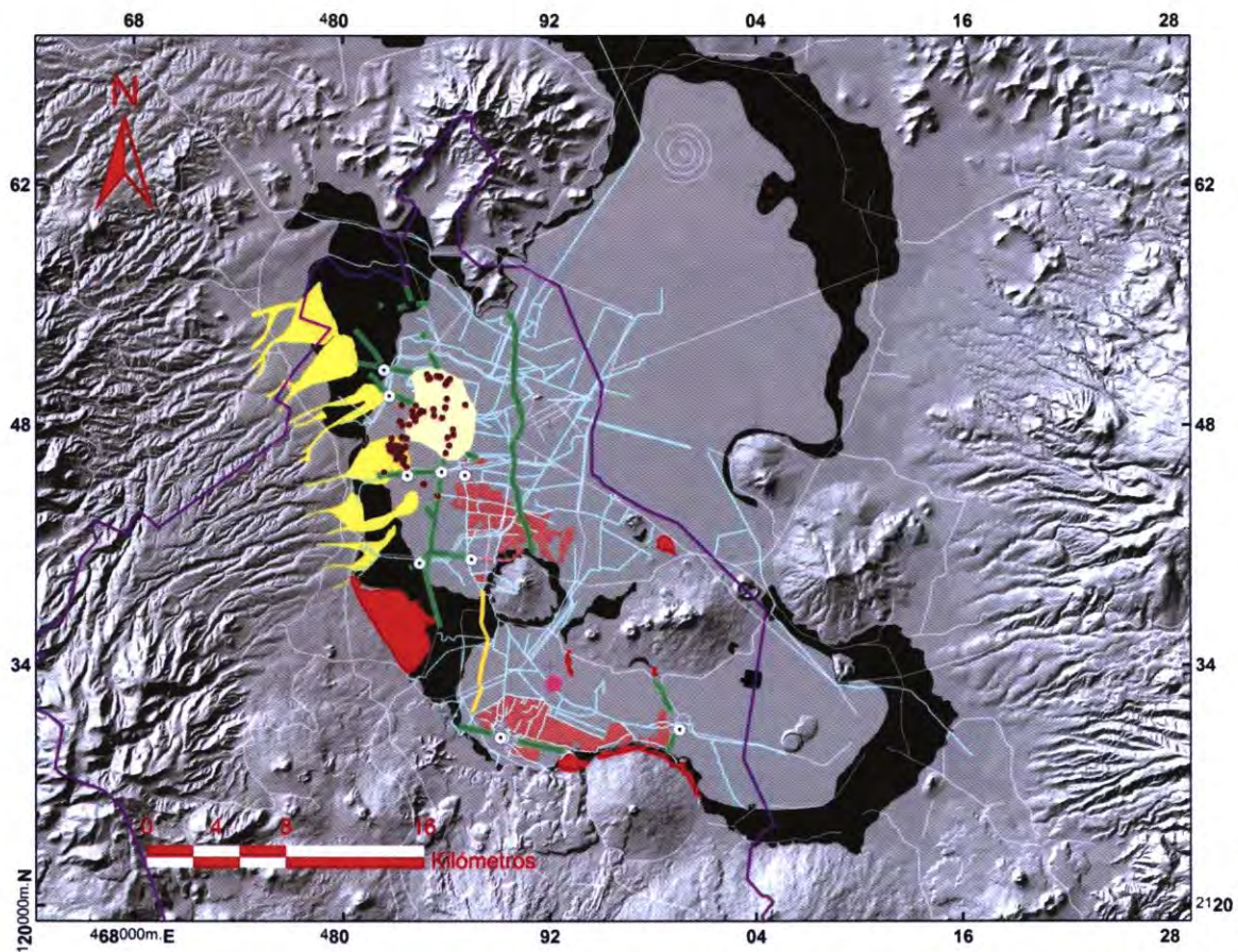
Fig. 18. Trazo del proyecto (amarillo pálido) bajo el contexto de las anomalías geotécnicas.
