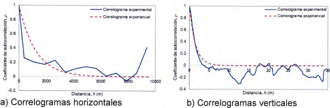
Fig. 15. Modelos de correlación espacial del contenido de agua.
