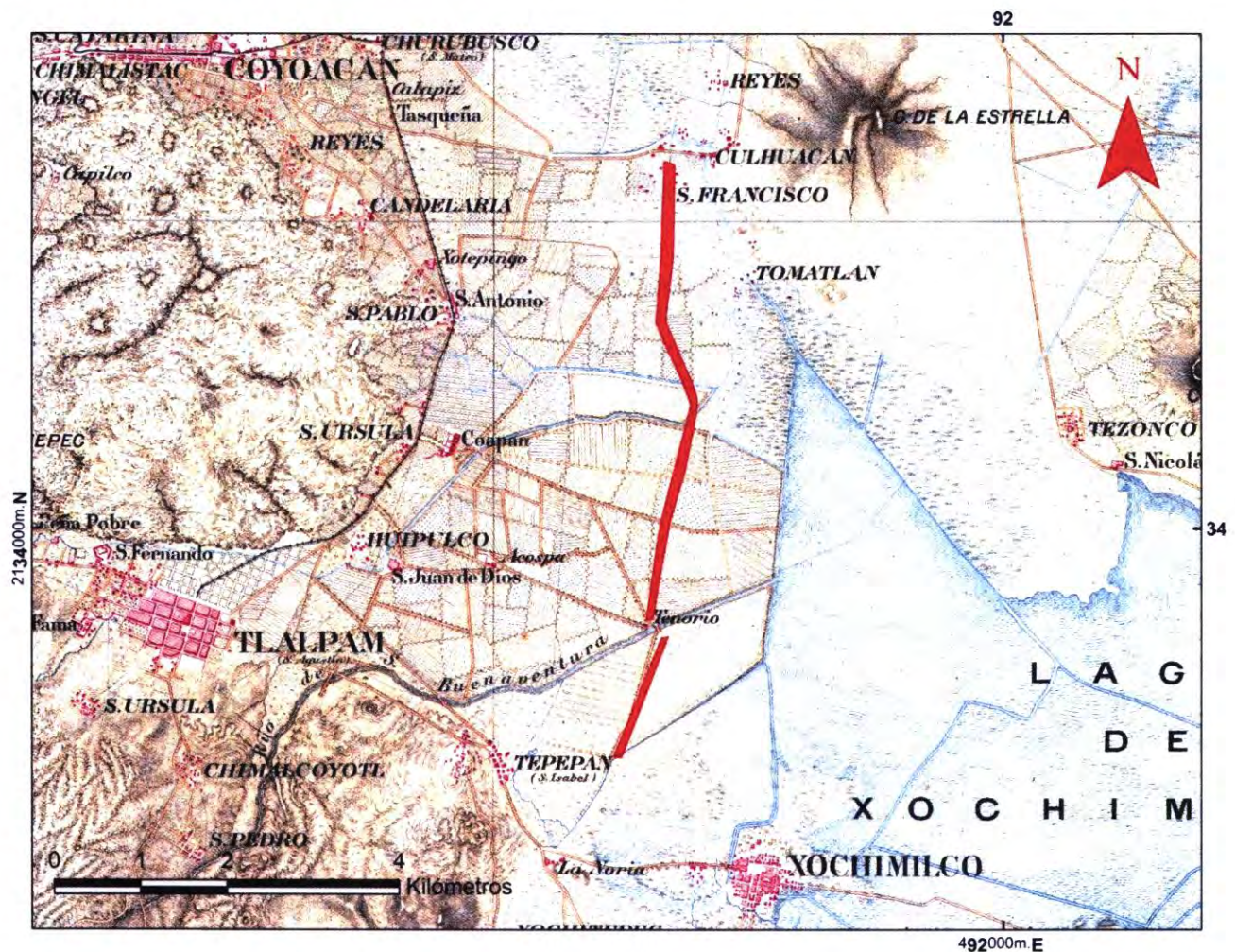
Fig. 3. Trazo del METROBÚS bajo el contexto de 1899, Manuel Fernández Leal.
