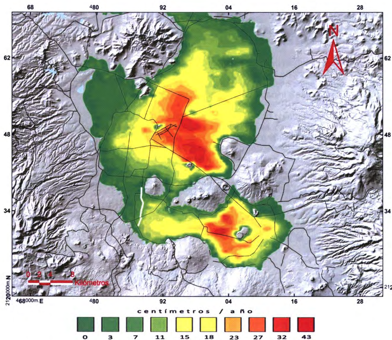
Fig. 20. Distribución espacial de las velocidades de hundimiento (1999 – 2008).
