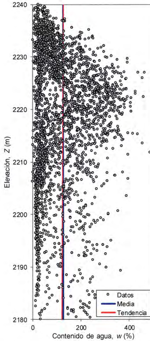
Fig. 14. Distribución de los datos en la zona de estudio a lo largo de la profundidad Z.
