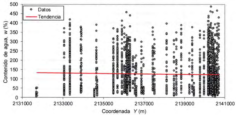
Fig. 13. Distribución de los datos en la zona de estudio a lo largo de la coordenada Y.
