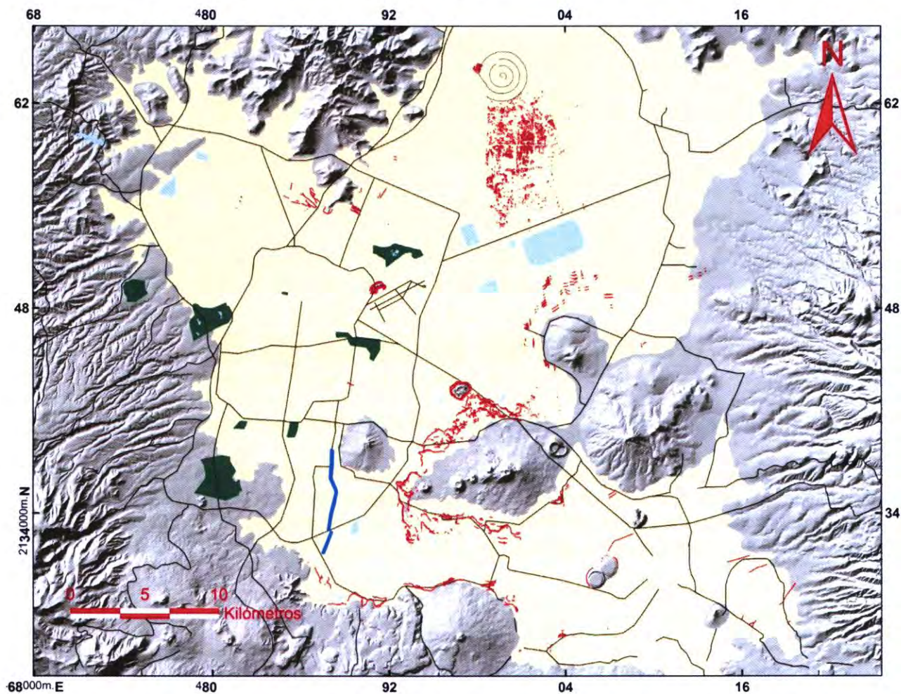
Fig. 21. Trazo del proyecto del METROBÚS bajo el contexto del fenómeno del agrietamiento.
