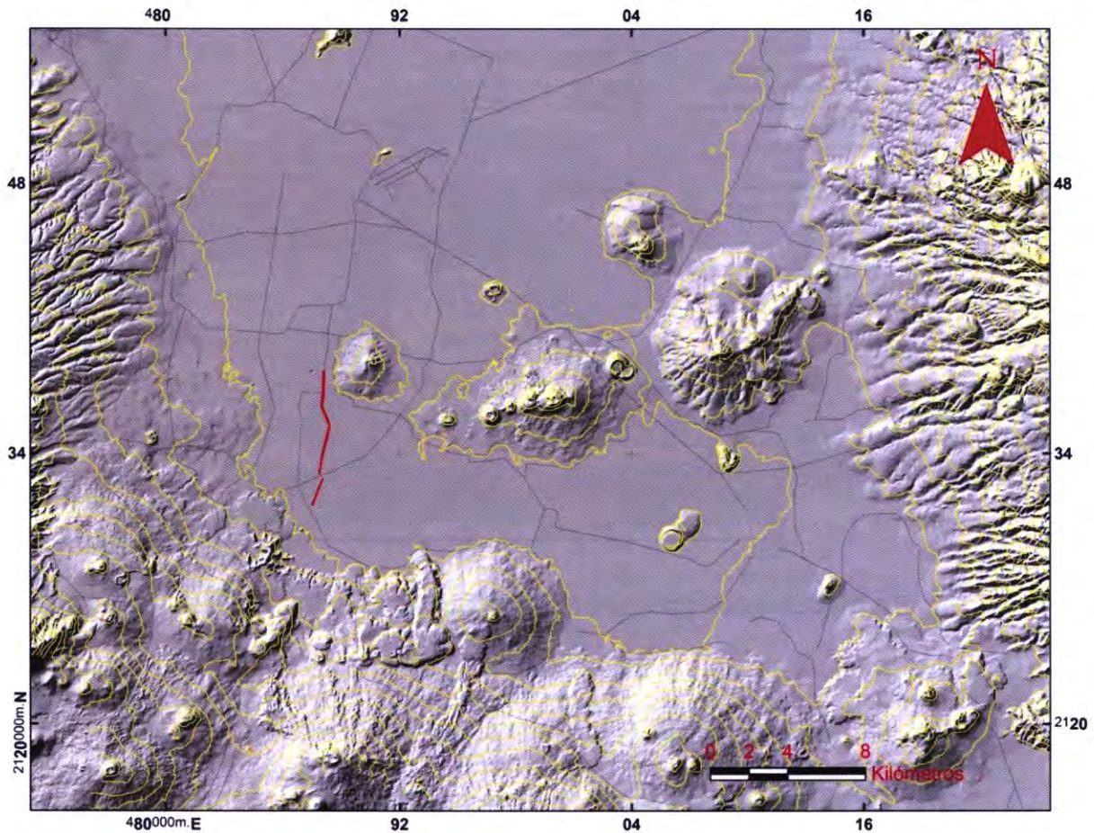
Fig. 4. Trazo del METROBÚS bajo el contexto del Modelo de Relieve Sombreado.
