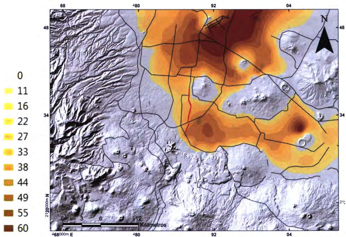
Fig. 10. Trazo del proyecto bajo el contexto de espesor de suelos blandos en metros.
