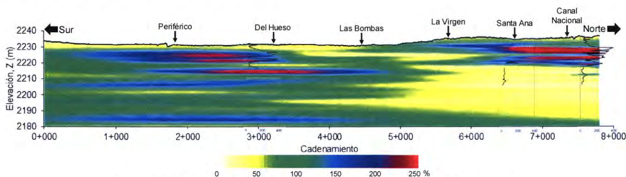
a) Sección transversal del contenido de agua estimado, w (%).
