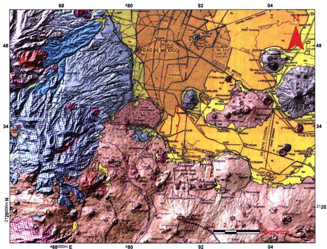
Fig. 6. Trazo del METROBÚS bajo el contexto de la Geología regional, (Mooser et al. 1996).
