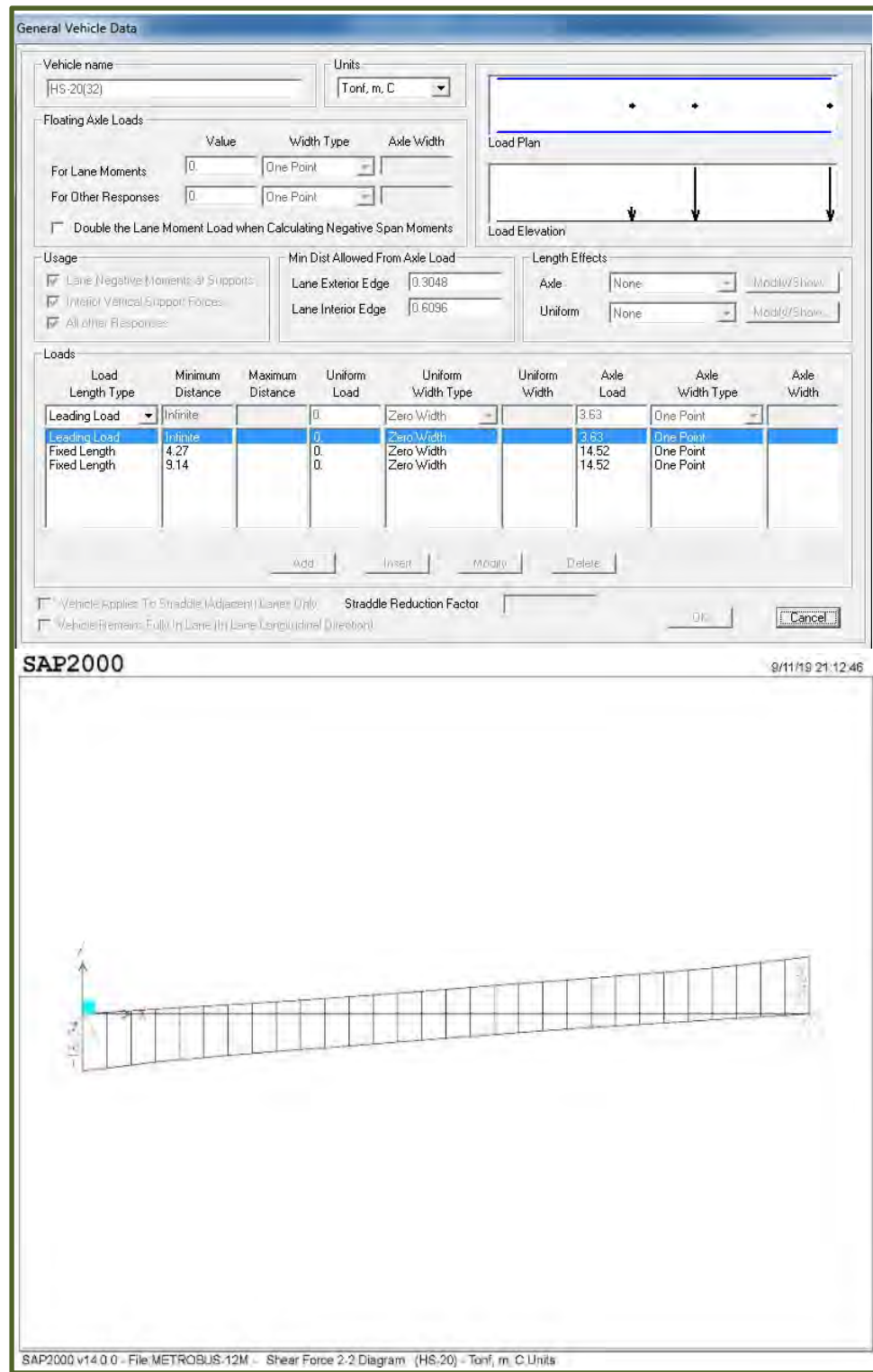
Figura No. 33.- Captura de información en programa SAP-2000 del camión HS-20 y resultado de la fuerza cortante por efecto de Línea de Influencia en 12.40 m.
