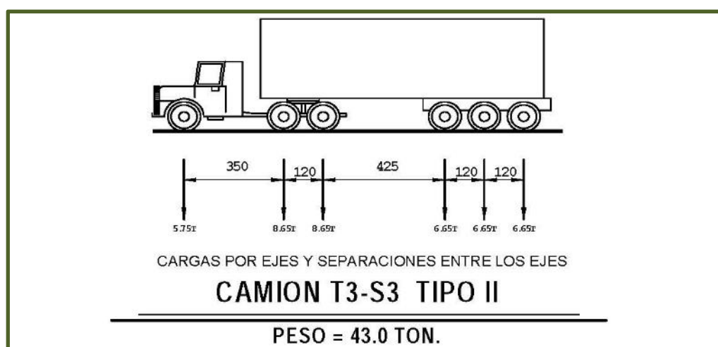
Figura No. 12.- Características de dimensiones y cargas para camiones tipo T3-S2-R4 y T3-S3, Tipo II.
