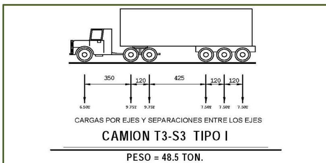
Figura No. 11.- Características de dimensiones y cargas para camiones tipo T3-S2-R4 y T3-S3, Tipo I.
