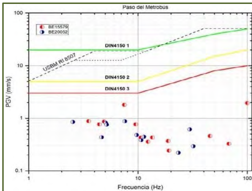
Figura No. 28.- Resumen de las observaciones de medición de ruido sísmico inducido por el paso del Metrobús.
