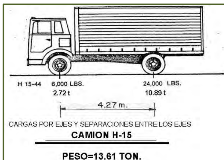
Figura No. 15.- Características de dimensiones y cargas para camión tipo H-15.
