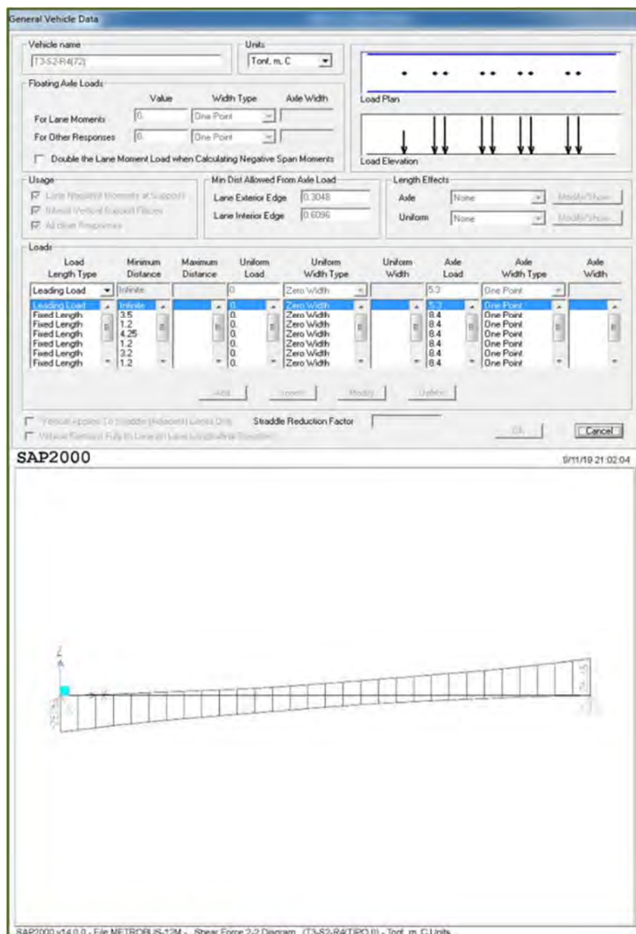
Figura No. 29.- Captura de información en programa SAP-2000 del camión T3-S2-R4 (TIPO I) y resultado de la fuerza cortante por efecto de Línea de Influencia en 12.40 m.
