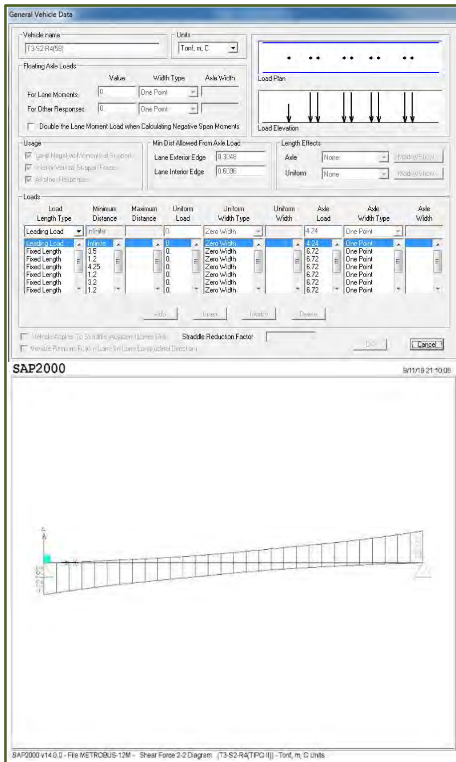
Figura No. 31.- Captura de información en programa SAP-2000 del camión T3-S2-R4 (TIPO II) y resultado de la fuerza cortante por efecto de Línea de Influencia en 12.40 m.
