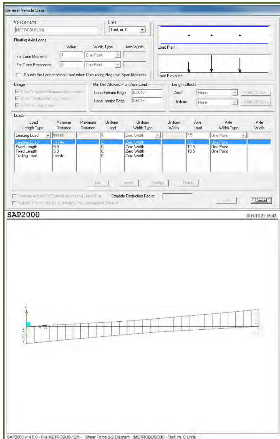
Figura No. 36.- Captura de información en programa SAP-2000 del Metrobús Articulado y resultado de la fuerza cortante por efecto de Línea de Influencia en 12.40 m.
