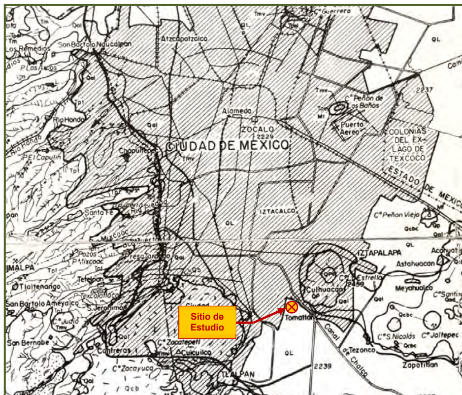
Figura No. 5.- Levantamiento geológico, Federico Mooser año 1956.
