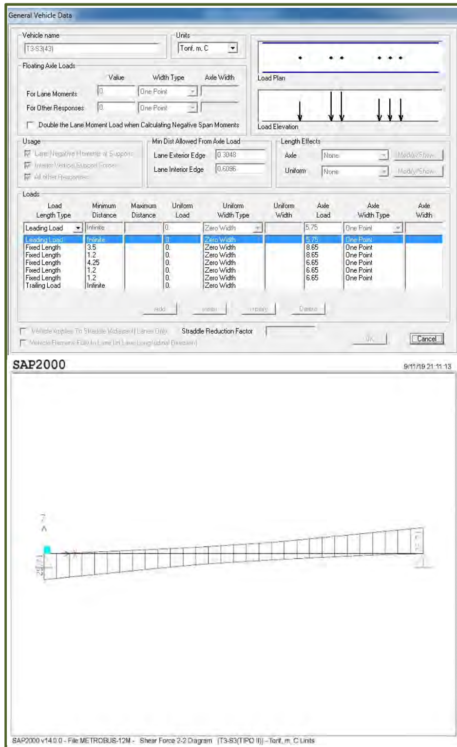
Figura No. 32.- Captura de información en programa SAP-2000 del camión T3-S3 (TIPO II) y resultado de la fuerza cortante por efecto de Línea de Influencia en 12.40 m.
