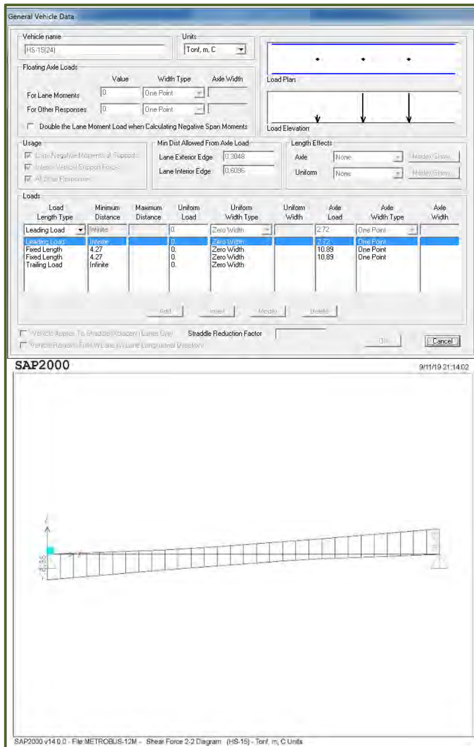
Figura No. 34.- Captura de información en programa SAP-2000 del camión HS-15 y resultado de la fuerza cortante por efecto de Línea de Influencia en 12.40 m.
