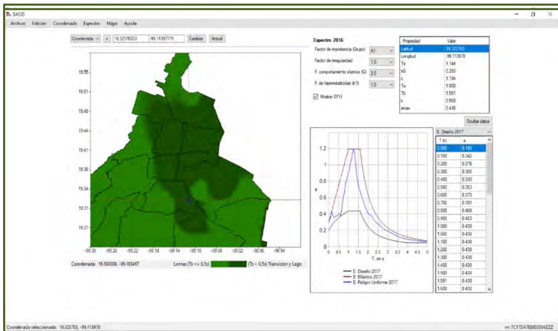
Figura No. 9.- Espectro para diseño sísmico para la estación La Virgen, NTC-Sismo CDMX, año 2017.
