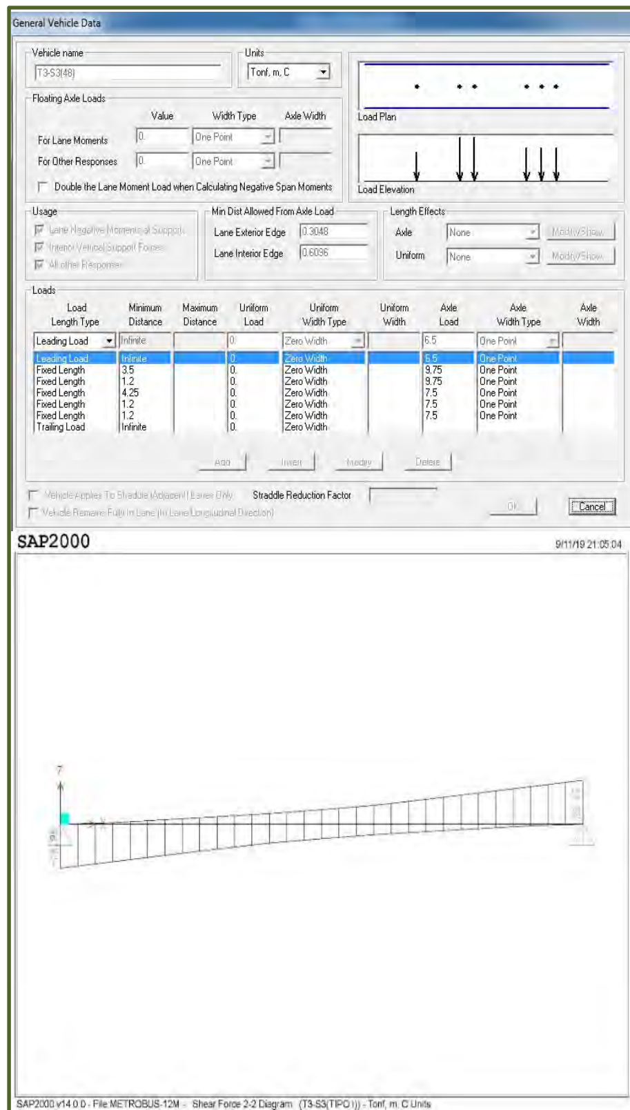
Figura No. 30.- Captura de información en programa SAP-2000 del camión T3-S3 (TIPO I) y resultado de la fuerza cortante por efecto de Línea de Influencia en 12.40 m.
