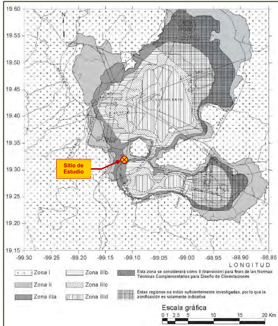
Figura No. 7.- Zonificación sísmica, NTC-Diseño Cimentaciones GDF, año 2004.
