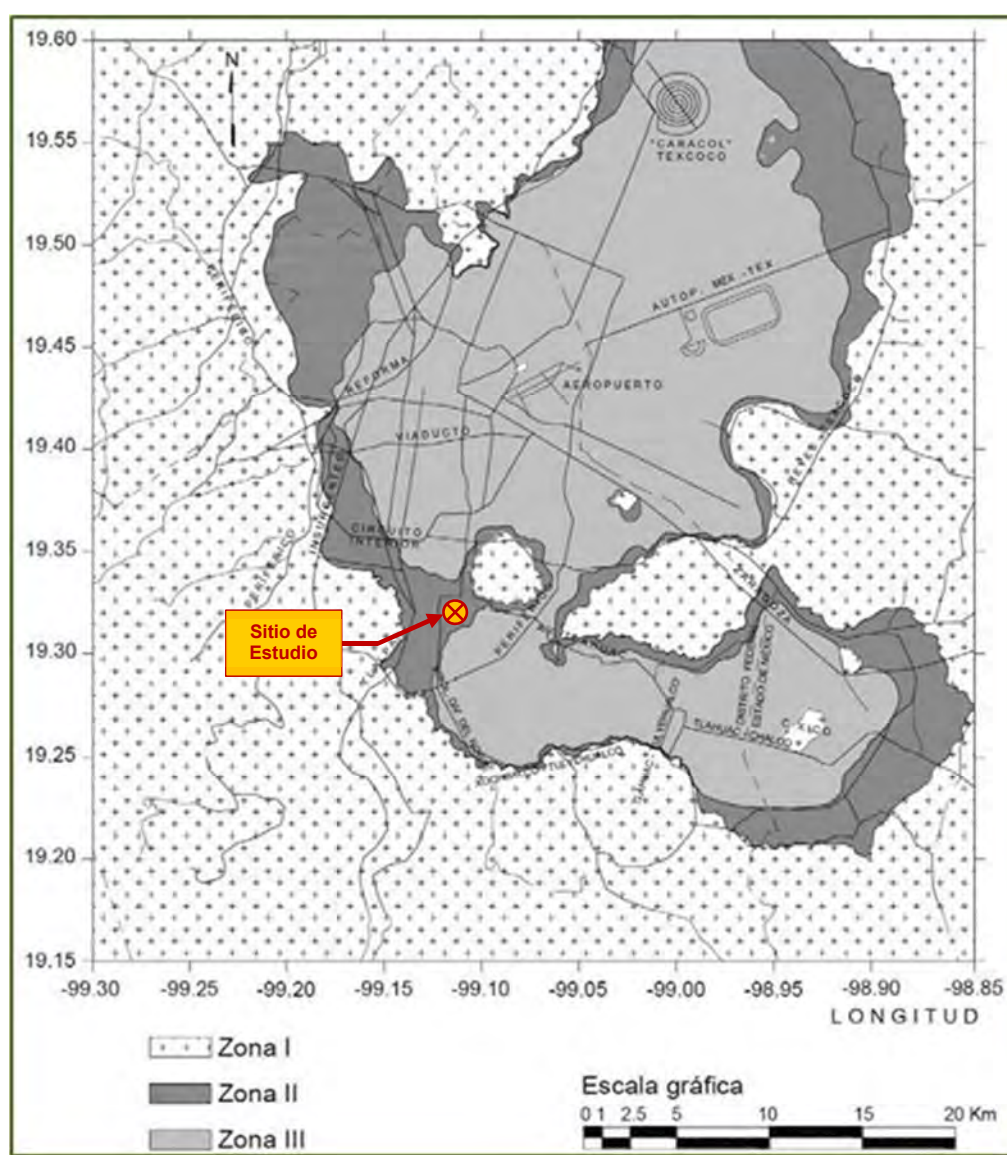
Figura No. 3.- Zonificación geotécnica, NTC-Diseño Cimentaciones CDMX, año 2017.
