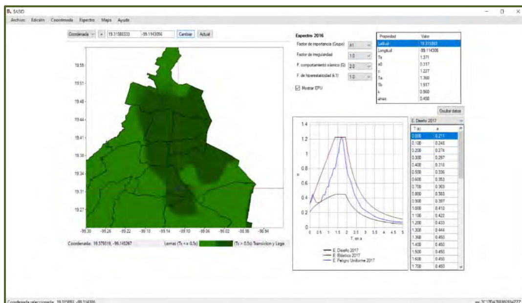
Figura No. 10.- Espectro para diseño sísmico para la estación Tepetlapa, NTC-Sismo CDMX, año 2017.
