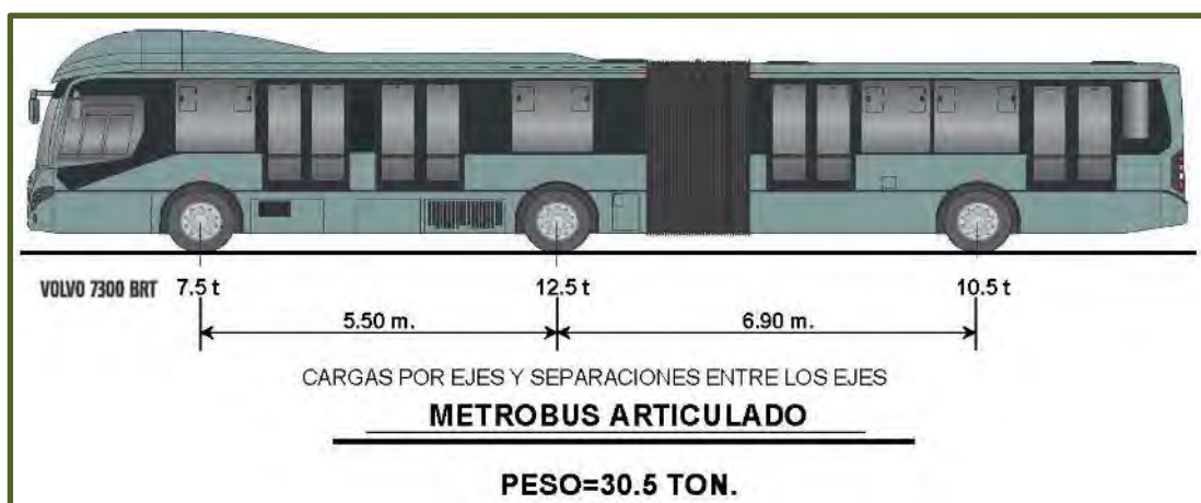
Figura No. 16.- Características de dimensiones y cargas para Metrobús articulado, marca VOLVO, modelo 7300 BRT.
