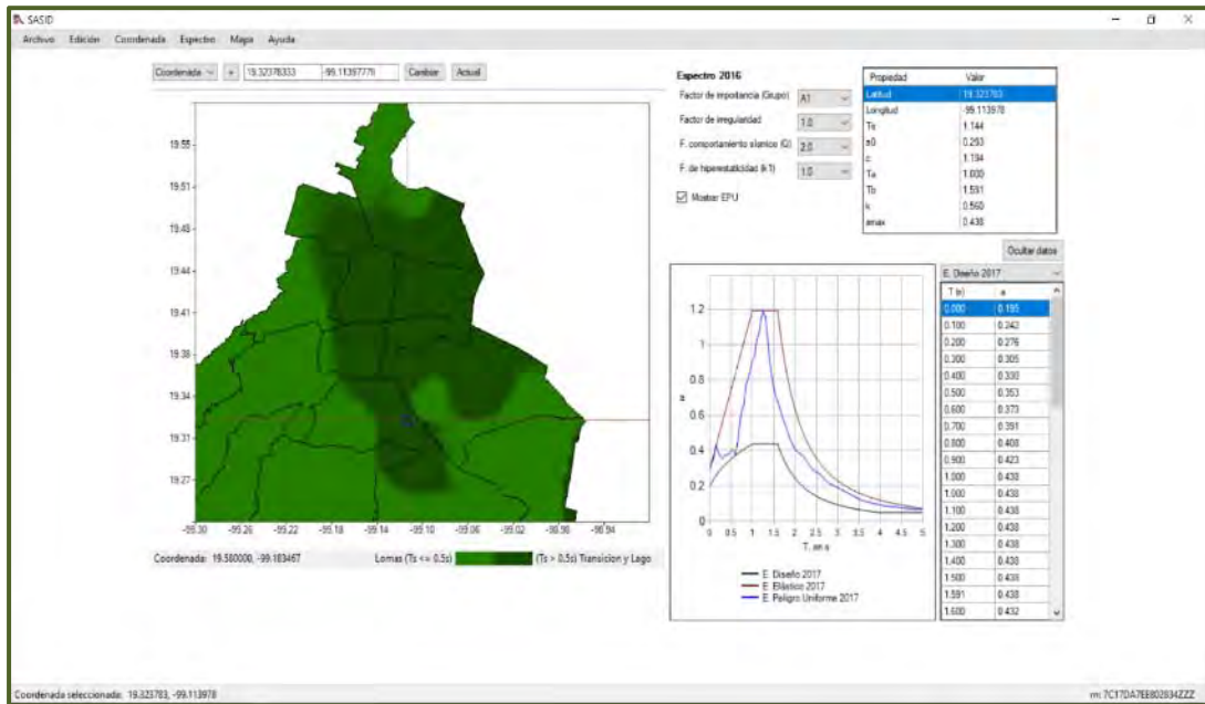
Figura No. 8.- Espectro para diseño sísmico para la estación Manuela Sáenz, NTC-Sismo CDMX, año 2017.
