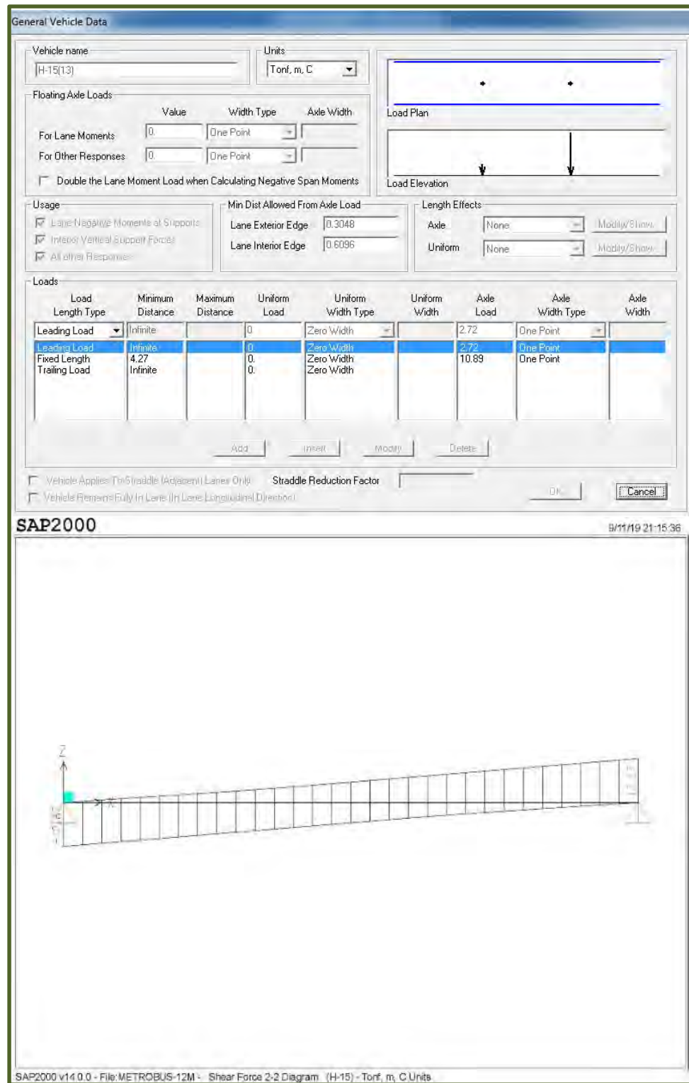
Figura No. 35.- Captura de información en programa SAP-2000 del camión H-15 y resultado de la fuerza cortante por efecto de Línea de Influencia en 12.40 m.
